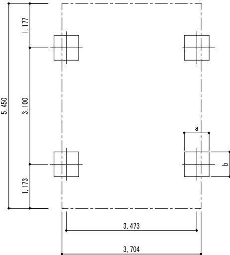
■基礎配置図
